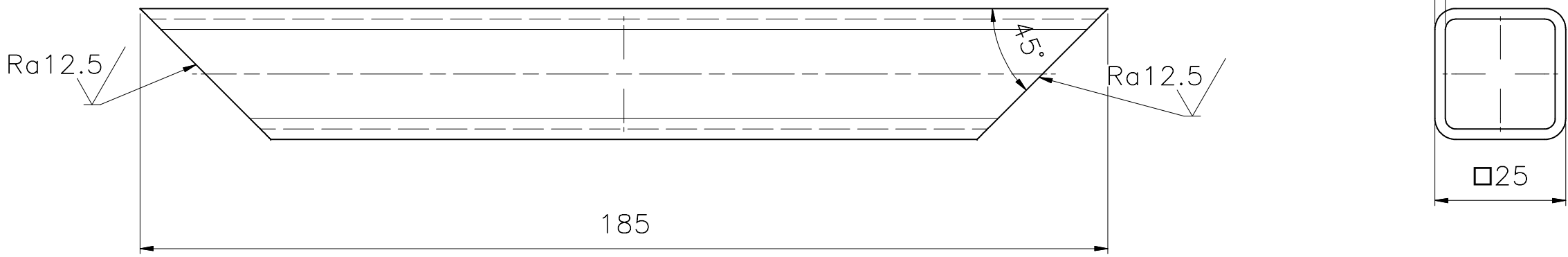
Item no.4 ( 1 : 1 )
