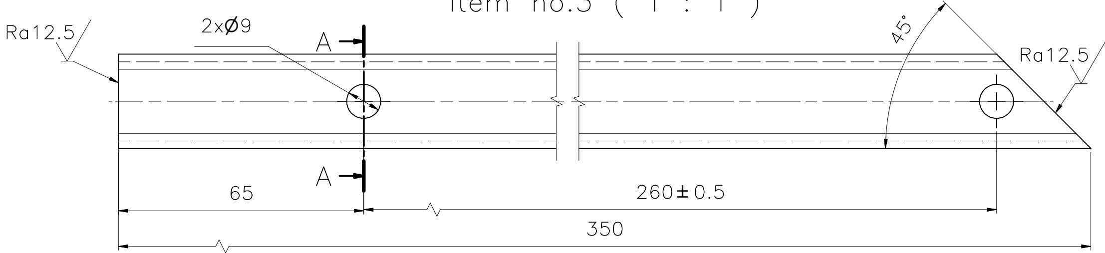
Item no.3 ( 1 : 1 )
